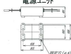
電源ユニット
