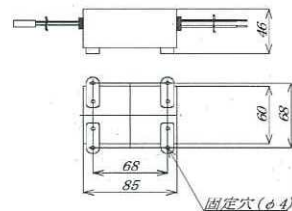
電源ユニット
