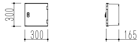
制御ボックス (防水仕様)
