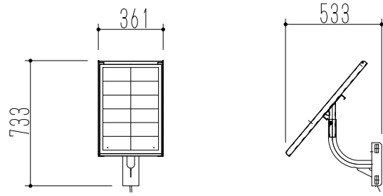
太陽電池
